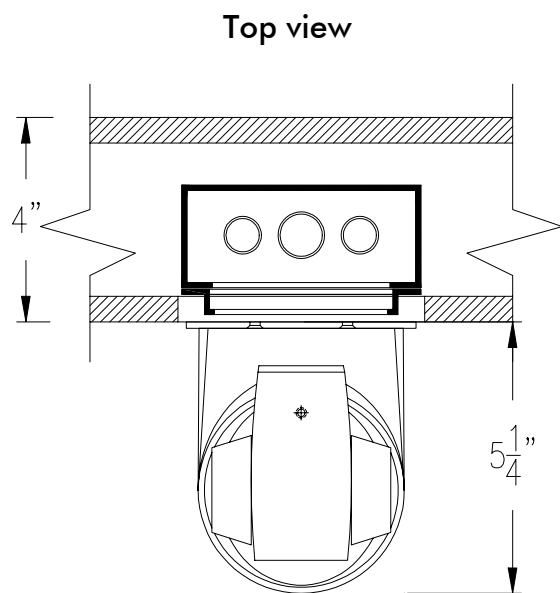
Head End module
