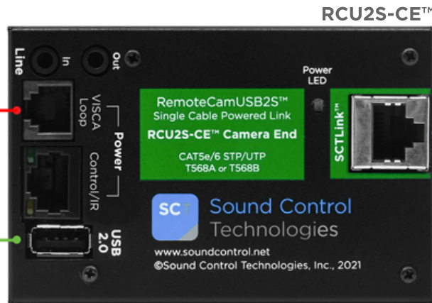
RCU2S-CE™
